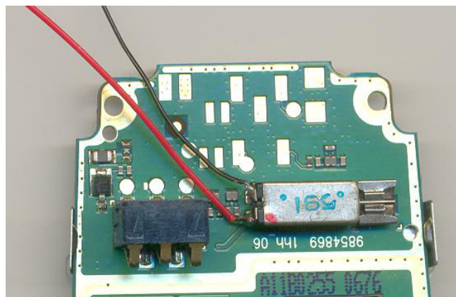
Abb. 4–11 Der Vibrationsmotor ist meist leicht zu identifizieren und an die beiden Kontakte lassen sich einfach zwei Kabel anlöten.
