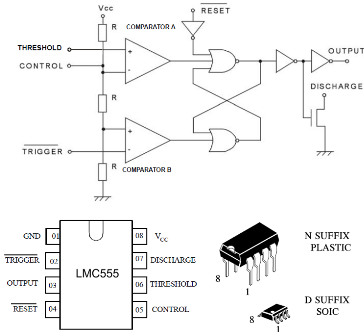
Abb. 4-13 Innenleben, Signale und Gehäuse des 555-Timerchips, dessen Kern aus einem RS-Flip-Flop mit einer davor geschalteten Komparatorschaltung besteht
