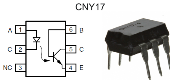
Abb. 4–12 Ein Optokoppler, wie der bekannte CNY17, enthält eine LED und einen Fototransistor, um zwei Schaltkreise elektrisch voneinander zu isolieren.
