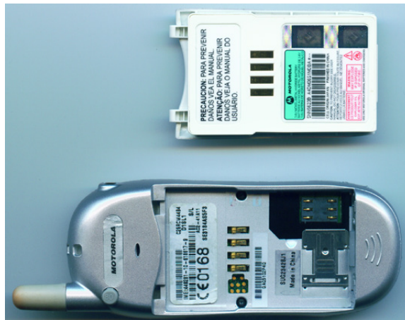
Abb. 4–2 Der NiMH-Akku ist mit dem Rückwanddeckel fest verbunden. Wenn er entfernt ist, gelangt man an die Schrauben für das Gehäuse.
