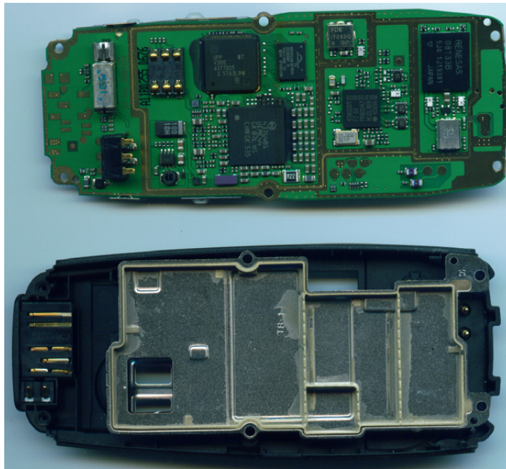
Abb. 4–6 Alle elektrischen Komponenten des Handys befinden sich auf der Platine.
