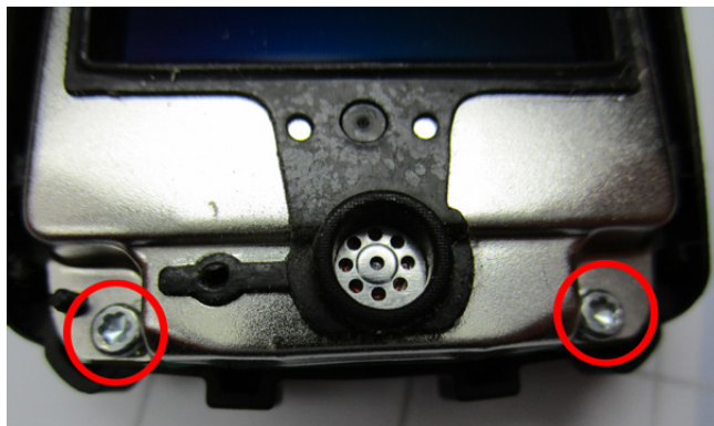
Abb. 4-4 Um das Handy weiter zerlegen zu können, sind beim Nokia-Modell von der Frontseite sechs dieser Torx-Schrauben zu lösen.
