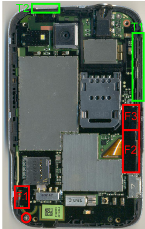
Abb. 4–10 Nach dem Lösen einer Schraube und von drei Foliengkabelverbindungen (F1-F3) lässt sich die Platine herausnehmen.
